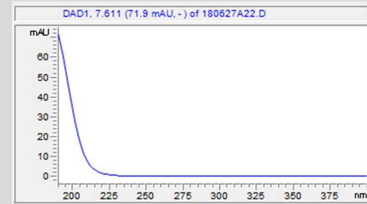
UV-Spektrum Hyaluronat
